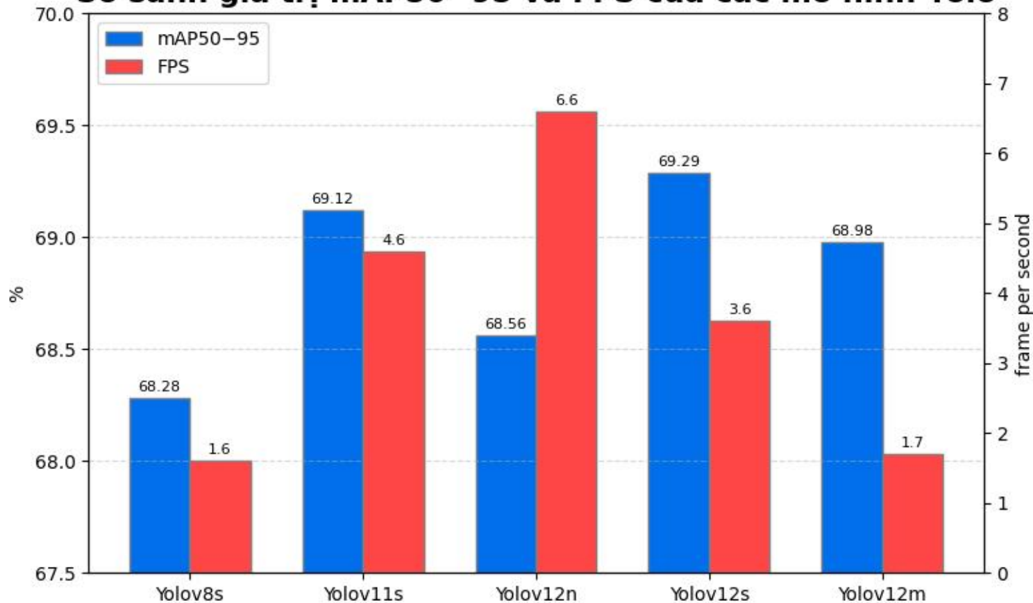
So sánh giá trị mAP50-95 và FPS của các mô hình Yolo
